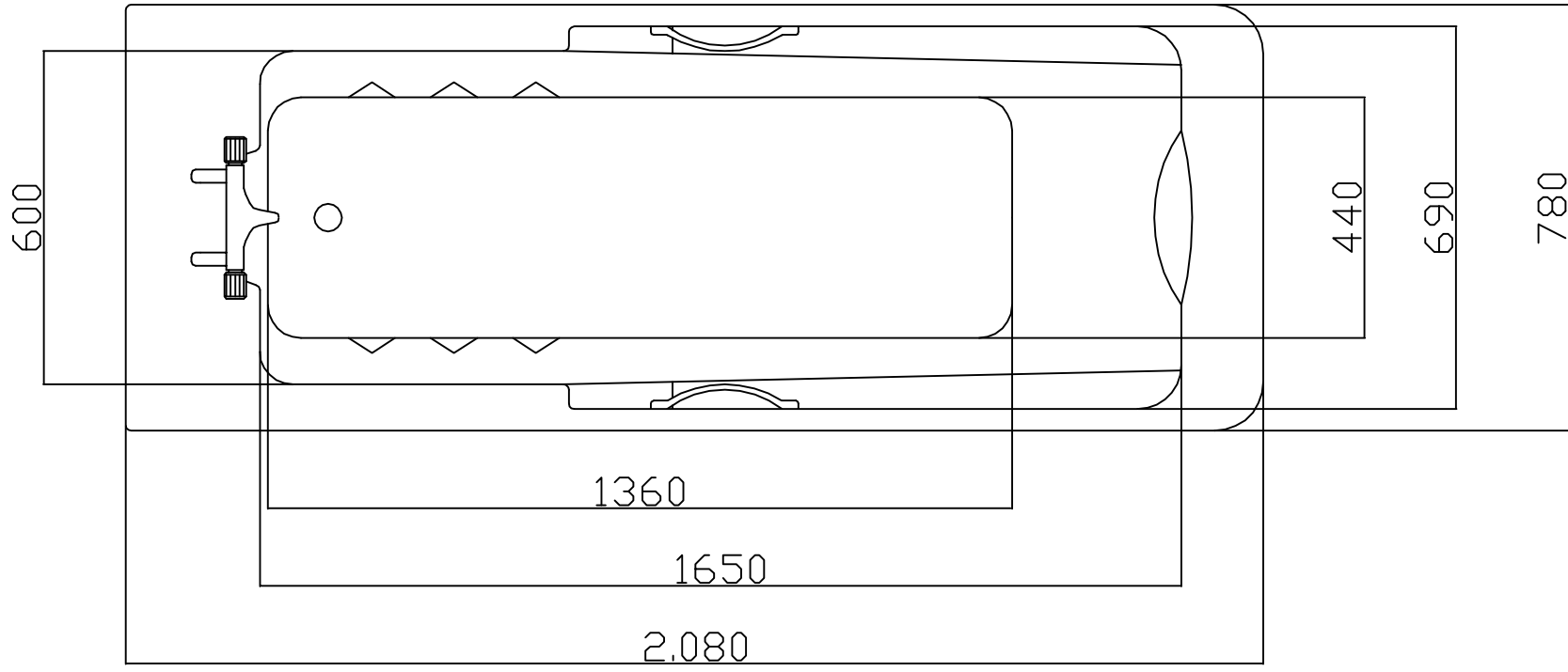
Innen- und Aussenmaße Hubwanne Comfortline II
